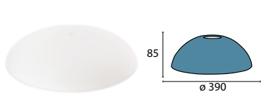
Glas 7-792/47 opal matt Ø 390 mm, H 85 mm opal matt Glaswandstärke 3 mm
