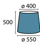
Schirm 12-4468 (f. Stl) Ø unten 550 mm, Ø oben 400 mm H 500 mm beige Material Stoff
