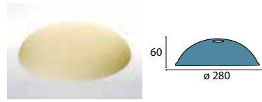
Glas 7-086 champ matt Ø 280 mm, H 60 mm champagne matt Öffnung 10 mm
