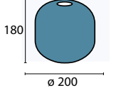
Glas 6-1818 rauch Ø 200 mm, H 180 mm rauch Öffnung 45 mm
