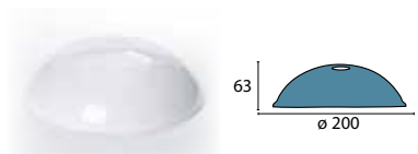
Glas 7-085 opal glänzend Ø 200 mm, H 63 mm opal glänzend Öffnung 11 mm
