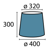
Schirm 12-1186 weiß Ø unten 400 mm, Ø oben 320 mm H 300 mm weiß Lampenhalter Höhe 65 mm
