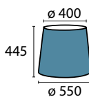
Schirm 12-4406 Dekor Ø unten 550 mm, Ø oben 400 mm H 445 mm creme Dekor Material Stoff
