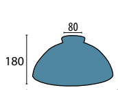
Glas 434 opal-matt/gold Ø 350 mm, H 180 mm opal matt Öffnung 42 mm Griffrand 80 mm
