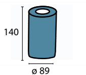
Glas 509 opal-matt Ø 89 mm, H 140 mm opal matt Öffnung 42 mm
