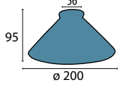
Glas 435 opal-matt/silber Ø 200 mm, H 95 mm opal matt Öffnung 42 mm Griffrand 56 mm
