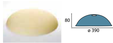
Glas 7-087 champ matt Ø 390 mm, H 80 mm champagne matt Öffnung 10 mm
