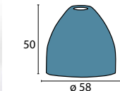
Glas 10-423 opal Ø 58 mm, H 50 mm opal matt Öffnung 21 mm, Fassung G9
