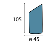
Glas 450 klar-matt Ø 45 mm, H 105 mm klar matt Öffnung 22 mm, Fassung G9
