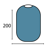
Glas 6-1816 opal Ø 140 mm, H 200 mm opal Öffnung 45 mm
