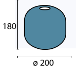
Glas 6-1818 grün Ø 200 mm, H 180 mm grün Öffnung 45 mm
