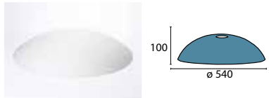
Glas 7-531/56 Ø 540 mm, H 100 mm opal matt Öffnung 12 mm
