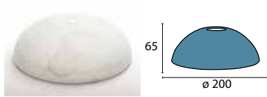
Glas 4-1136 opal Ø 200 mm, H 65 mm matt Öffnung 20 mm
