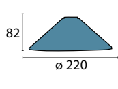
Glas 445 kobalt Ø 220 mm, H 82 mm blau Öffnung 30 mm
