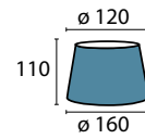
Schirm 4461 weiß Ø unten 160 mm, Ø oben 120 mm H 110 mm weiß Material Organza
