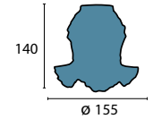
Glas 492 Ø 155 mm, H 140 mm klar matt Öffnung 51 mm
